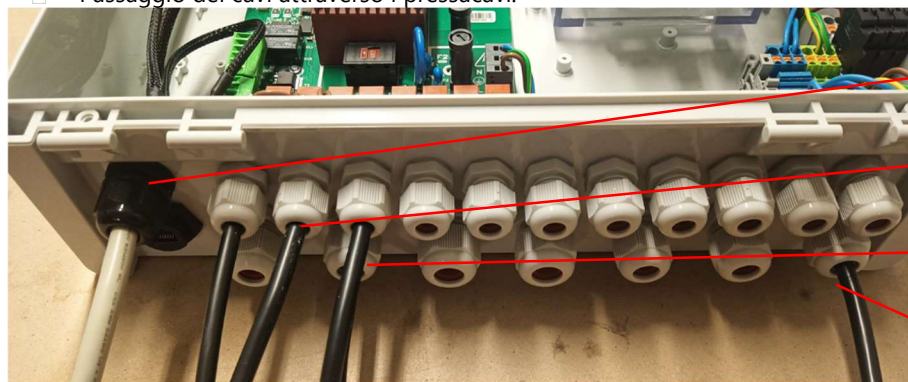
Figure 14 – Passaggio dei cavi attraverso i pressacavi
