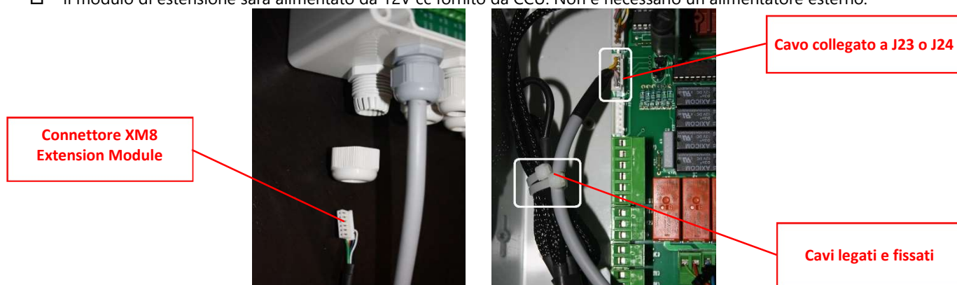
Figure 59 - Entrées de câbles
