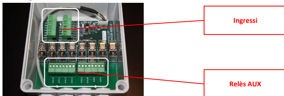
Figure 60 - Morsetti di collegamento
