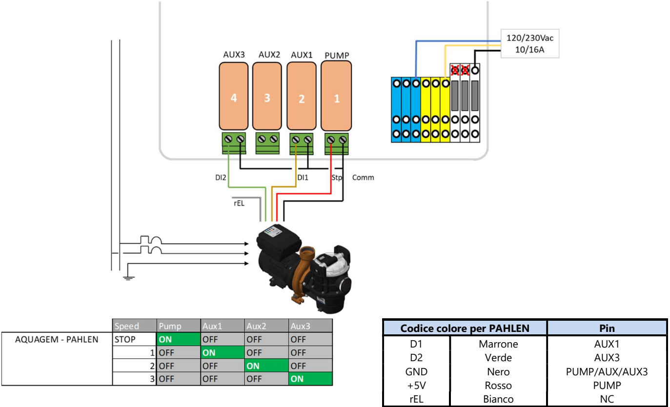
Figura 34– PAHLEN EcoVISE, EcoFloVISE
